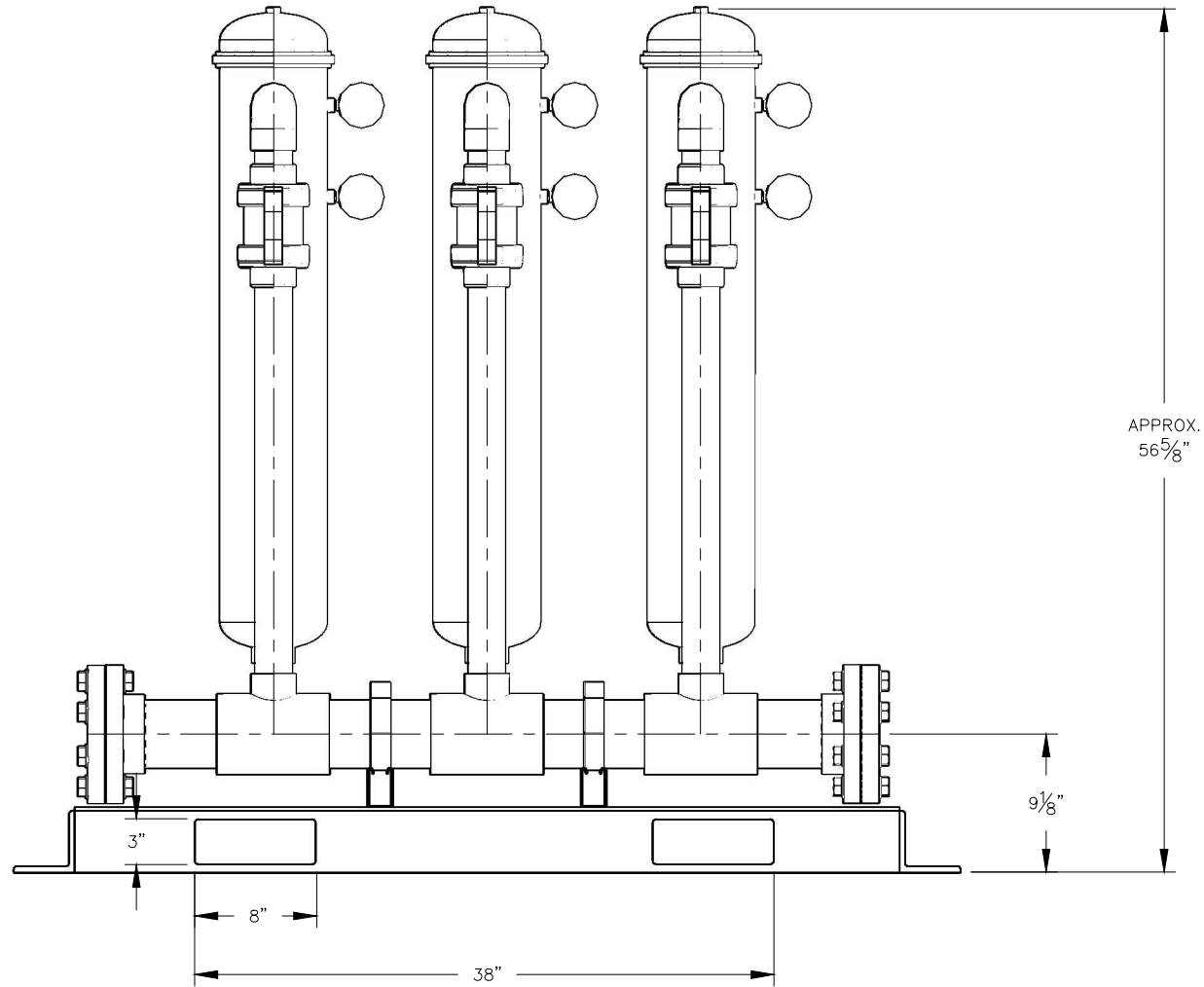
ELEVATION
