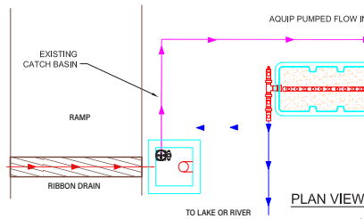
Aquip 10 - top view
