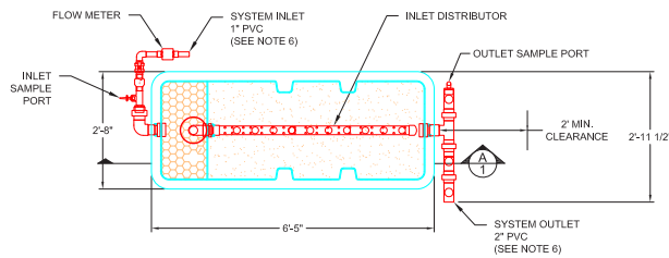
Aquip 10 - top view
