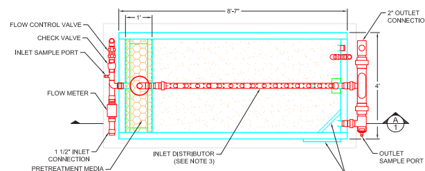
Aquip 25 - top view
