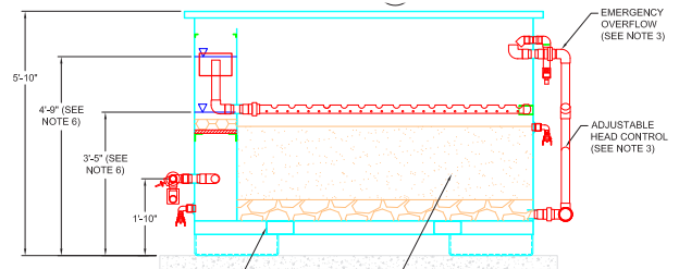
Aquip 25 - side view
