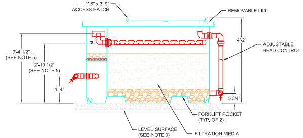
Aquip 10 - side view
